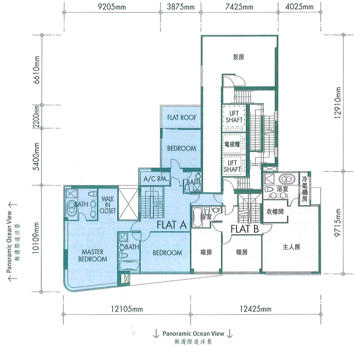
53/F ROOF PLAN 平面圖
